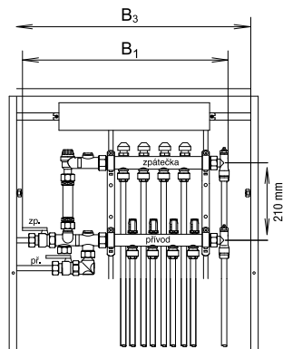
Napojení z boku doplňující díly 2 ks GT-AVR 1" 01732 1 ks GT-ASW 1" 04385
