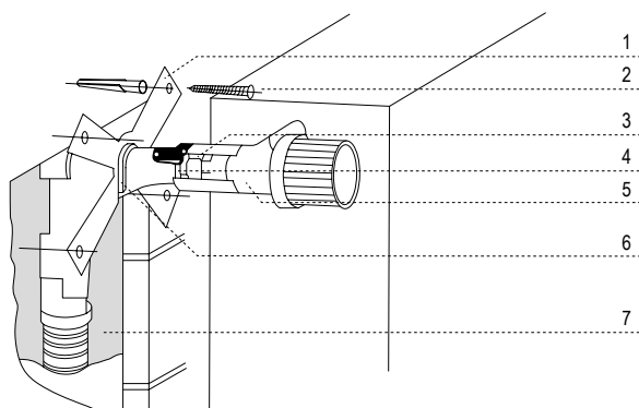
Detail C* Stěnové připojení
