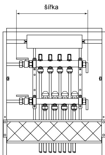
Detail A* Rozdělovač
