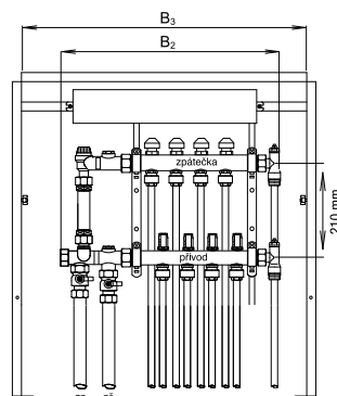
Napojení zespodu doplňující díly 2 ks GT-AVR 1" 01732
