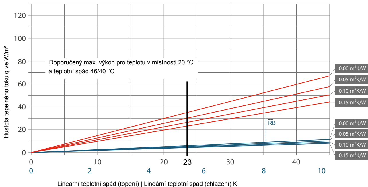
Diagram charakteristik vytápění a chlazení Gabotherm® Therm 25-10, 15x1,5, 16x2, RA = 334 mm
