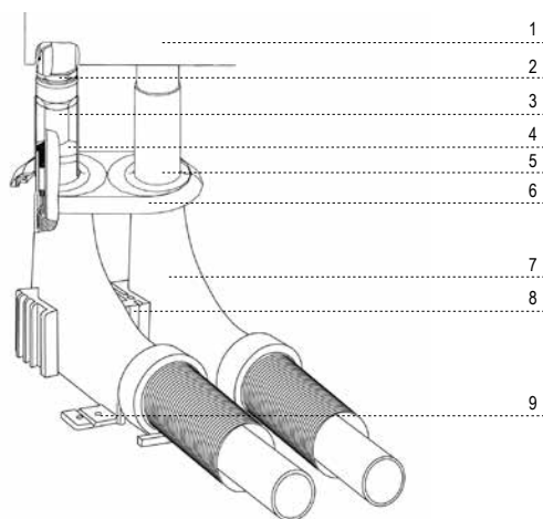
Detail B* Podlahové připojení
