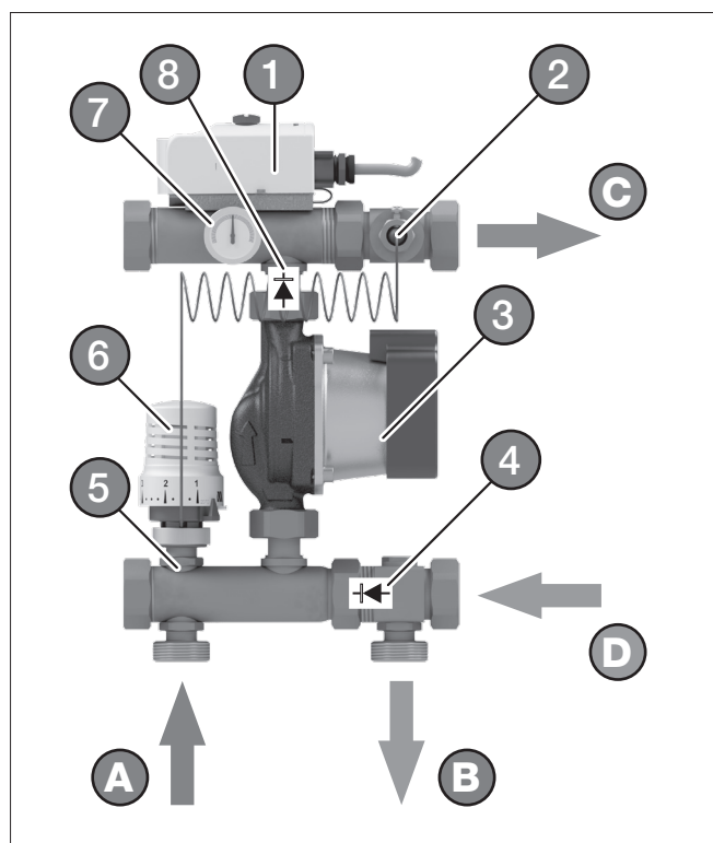
Obr. 3 – Přehled komponent
